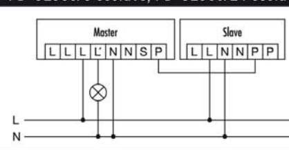
Branchement maître/esclave:
