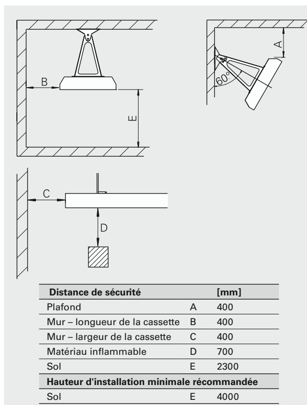
Fig. 1 : Distance de sécurité pour une installation fixe.
