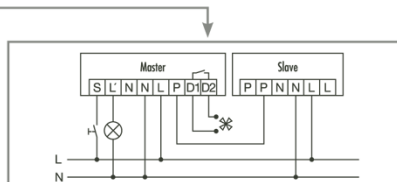
Branchement maître/esclave : l'appareil maître gère les dispositifs reliés selon les paramètres indiqués. Les appareils esclaves ne servent qu'à détecter une éventuelle présence et à envoyer une impulsion à l'appareil maître le cas échéant.
