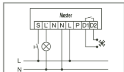
Installation standard + bouton permettant d'allumer ou d'éteindre l'éclairage manuellement si nécessaire.
