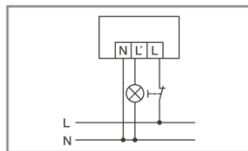
Installation standard avec possibilité d'allumage manuel.
